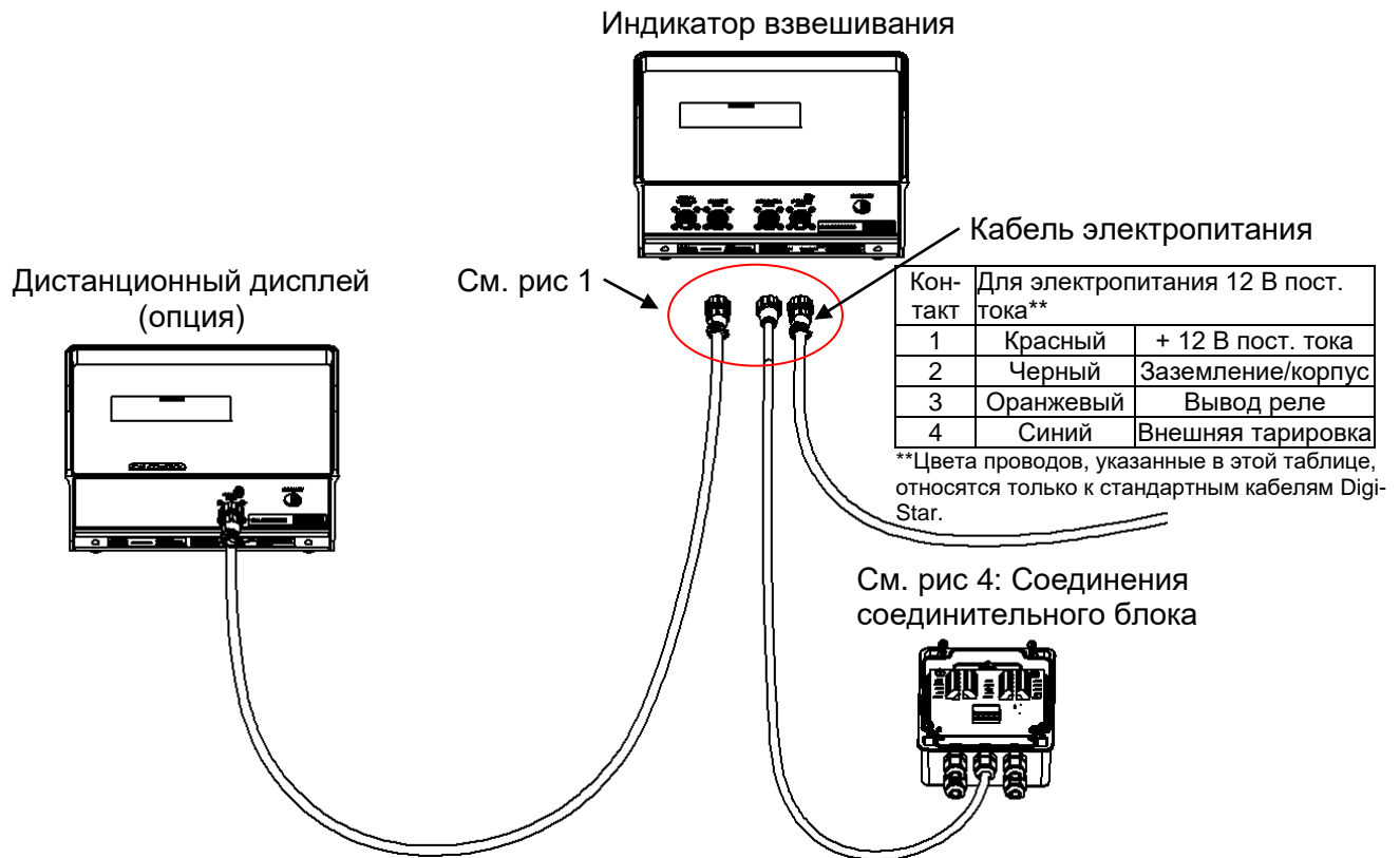
Рис. 2. Схема соединений индикатора взвешивания
